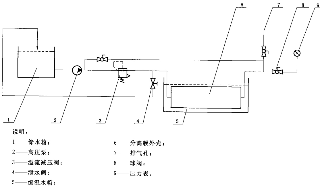
图 2 分离膜外壳循环水压渗漏试验原理图
