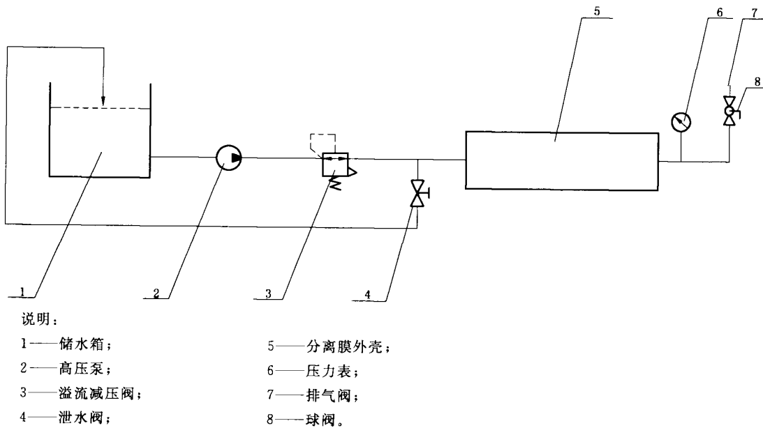
图 1 分离膜外壳静水压渗漏试验原理图
